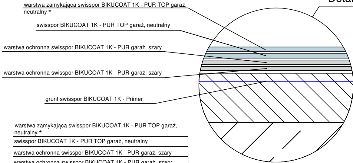
Detal A
